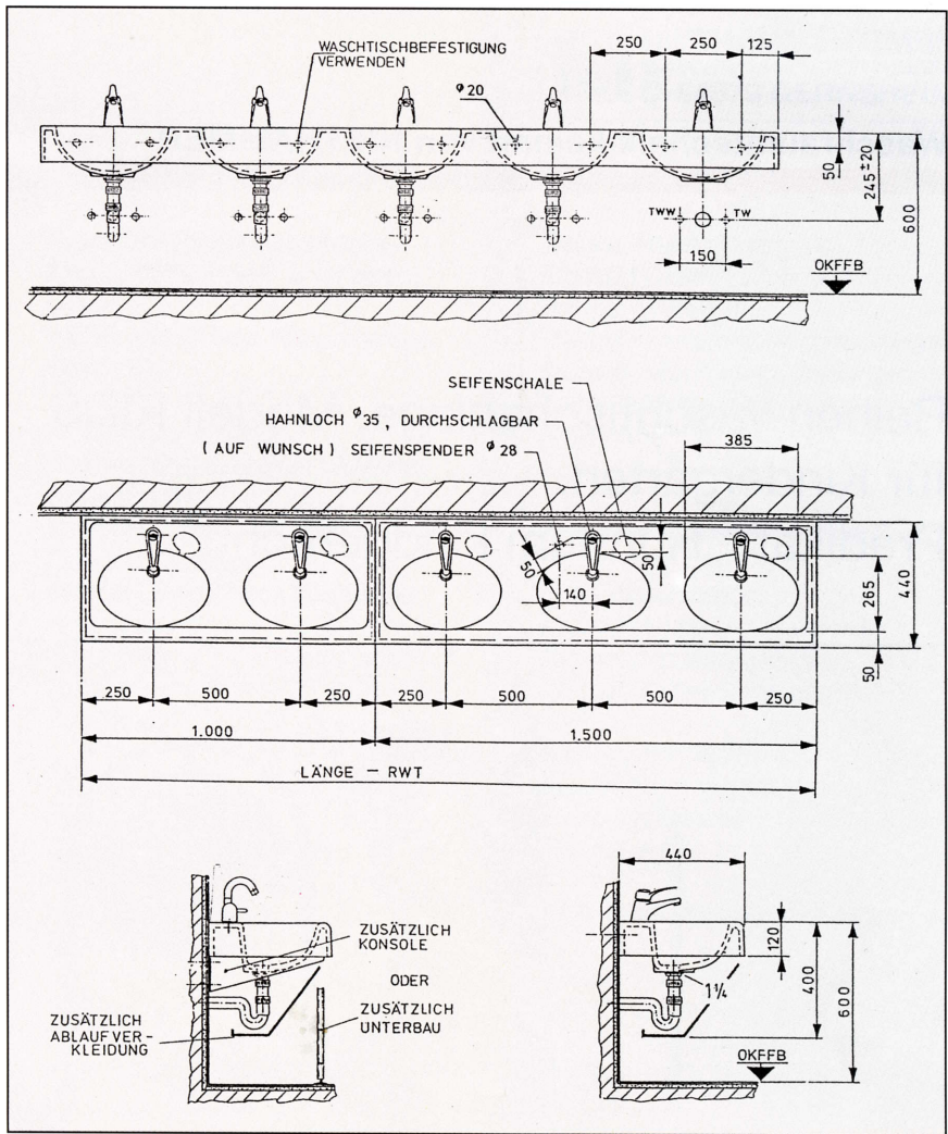
Planungsbeispiel einreihig, zur Wandmontage
